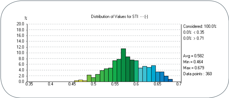
Abb. 3 STI-Verteilung mit allen Lautsprechern aktiv und allen Bereichen besetzt
