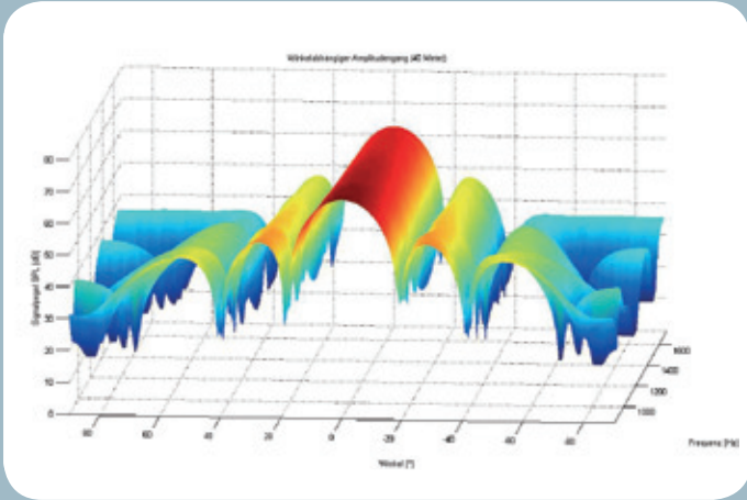
Abb. 1 Delay-Algorithmus / 1 Beam mit schmalem Öffnungswinkel
