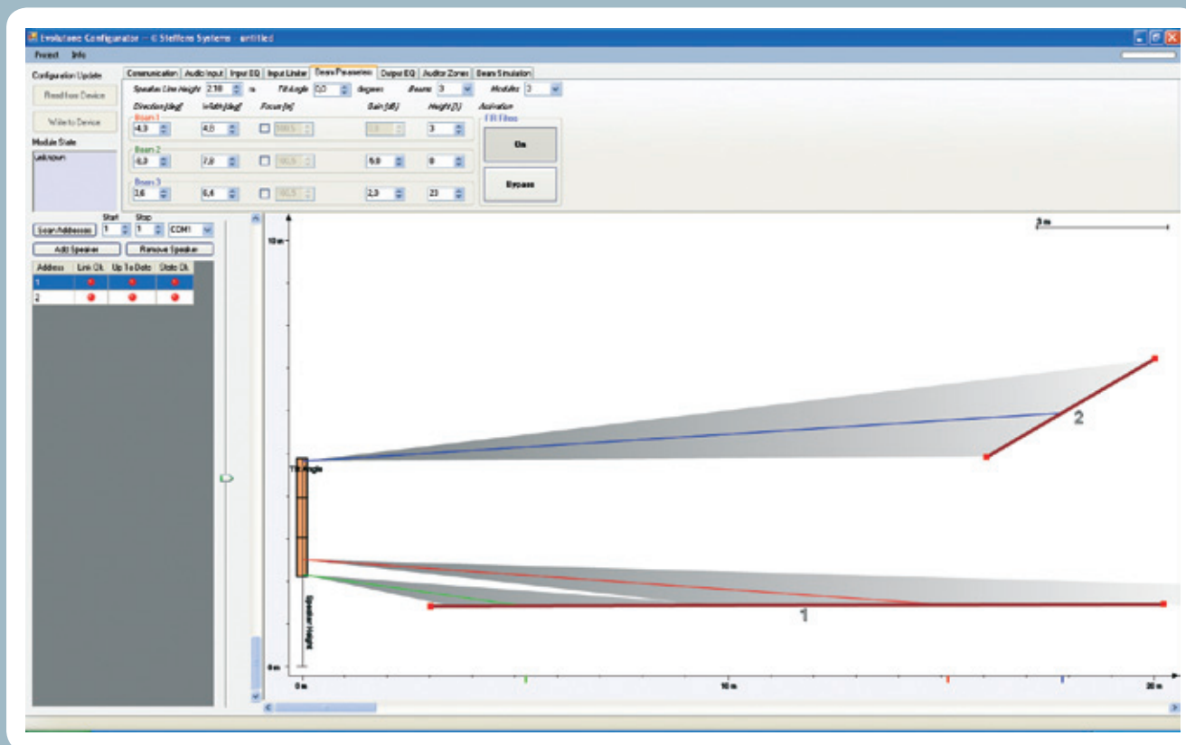
Abb. 1 evolutone 3-Beam / 3 unterschiedliche akustische Zentren
