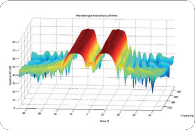
Abb. 4 evo-Algorithmus / 2 Beams mit schmalem Öffnungswinkel
