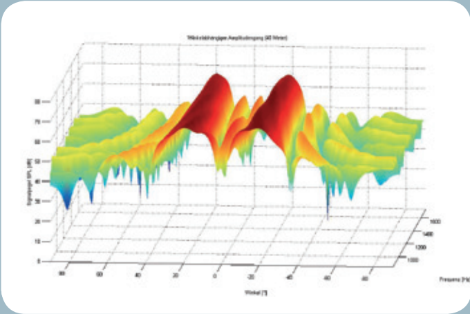
Abb. 2 Delay-Algorithmus / 2 Beams mit schmalem Öffnungswinkel
