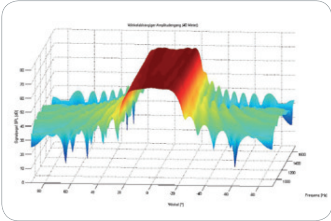
Abb. 3 evo-Algorithmus / 1 Beam mit schmalem Öffnungswinkel
